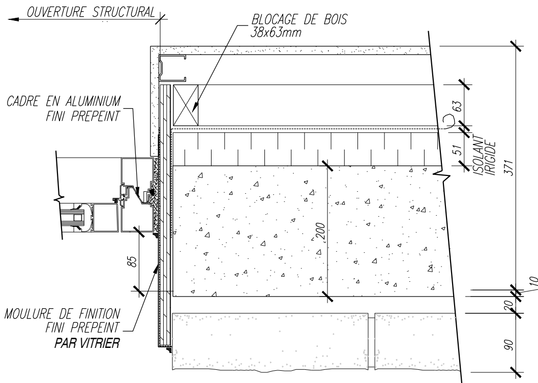
JAMBAGE D'UNE PORTE DOUBLE EN ALUMINIUM AU BETON
