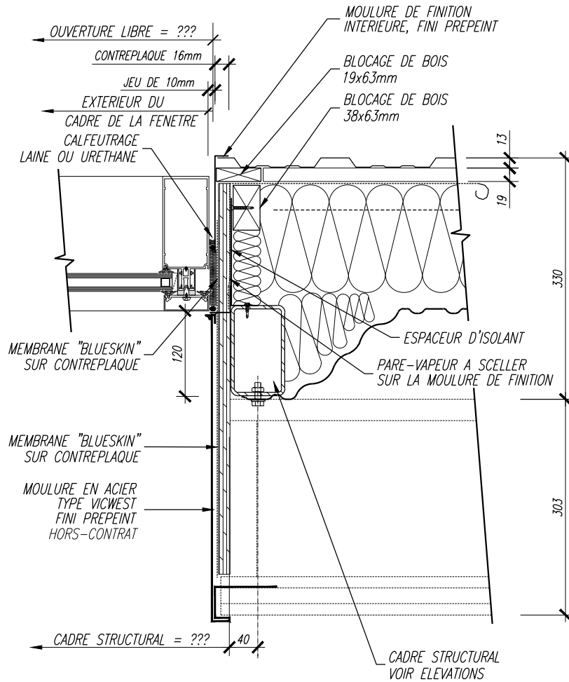
JAMBAGE D'UNE FENETRE EN ALUMINIUM
