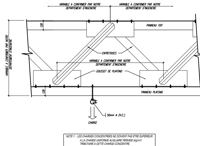
X 12 SUSPENSION APPAREILLAGE DE MECANIQUE 50 OU 64mm Ø PERPENDICULAIRE AU PANNEAU STRUCTURALE (COUPE LONGITUDINALE)
