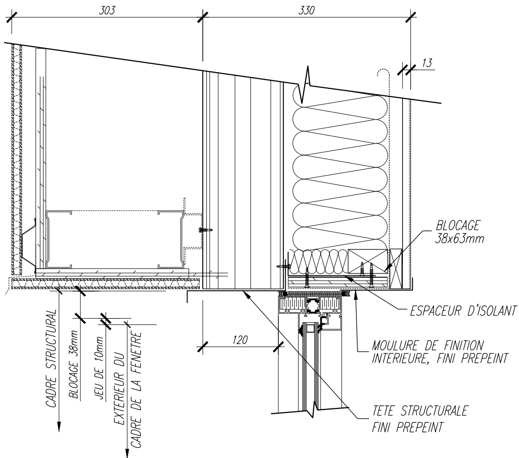
TETE D'UNE FENETRE EN ALUMINIUM
