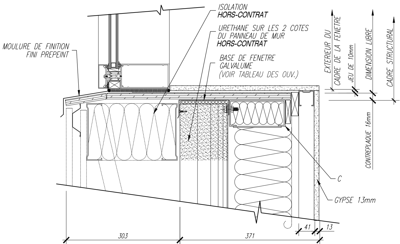
BASE D'UNE FENETRE EN ALUMINIUM
