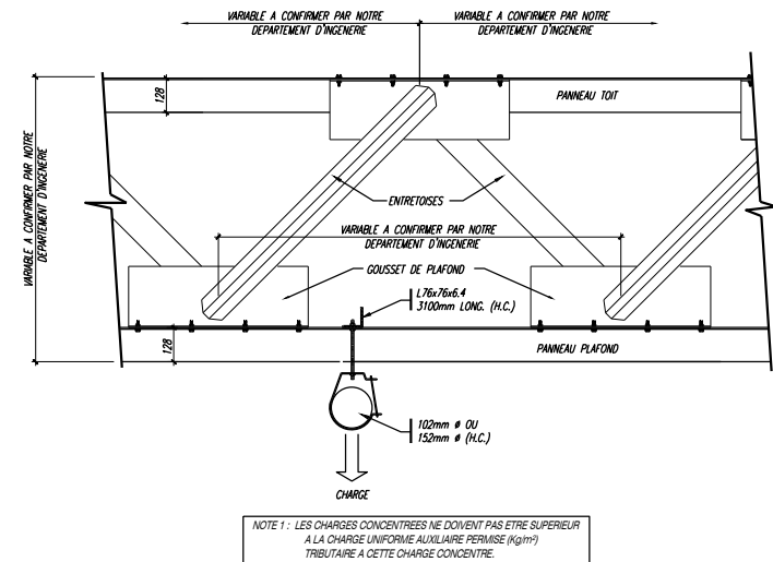
X X X SUSPENSION APPAREILLAGE DE MECANIQUE 102 OU 152mm Ø PERPENDICULAIRE AU PANNEAU STRUCTURALE (COUPE LONGITUDINALE)
