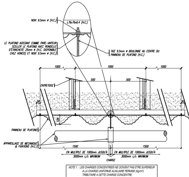
X X X SUSPENSION APPAREILLAGE DE MECANIQUE 102 OU 152mm Ø PERPENDICULAIRE AU PANNEAU STRUCTURALE (COUPE TRANSVERSALE)
