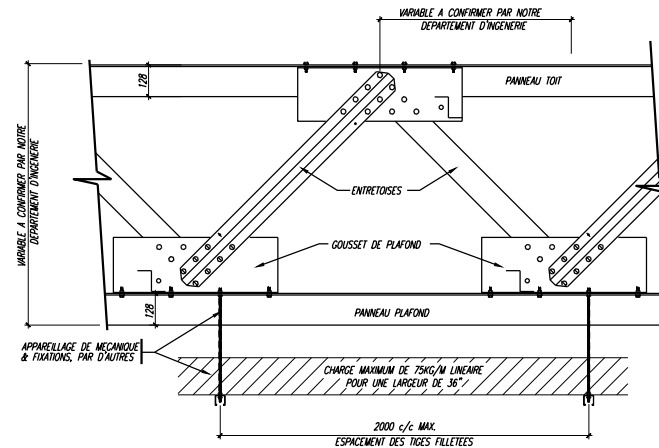
(X) SUSPENSION APPAREILLAGE DE MECANIQUE (Y) VIS-A-VIS LES GOUSSETS PLAFOND (Z) (COUPE LONGITUDINALE)
