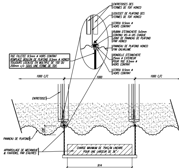
(X) SUSPENSION APPAREILLAGE DE MECANIQUE (Y) VIS-A-VIS LES GOUSSETS PLAFOND (Z) (COUPE TRANSVERSALE)
